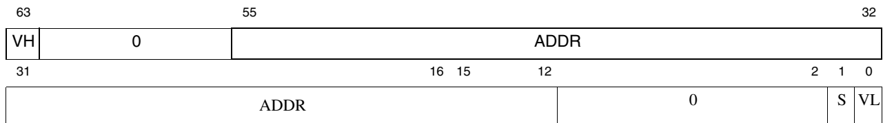
Figure 9.59 MAAR Register Format if PageGrain ELPA =1
